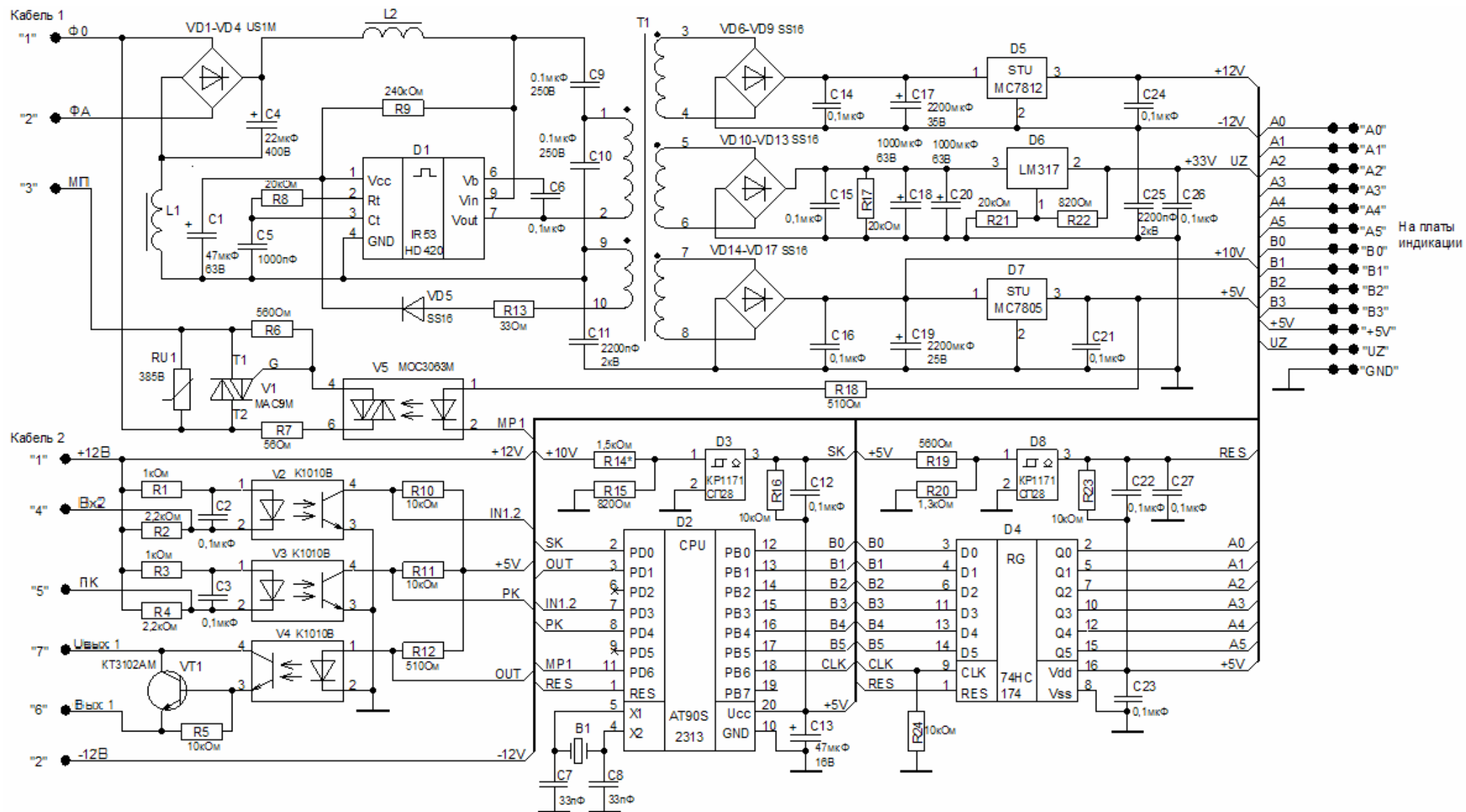
Фрагмент схемы электрической принципиальной устройства отсчетного ЭЦТ 1/5МА-4: входные и выходные цепи.
