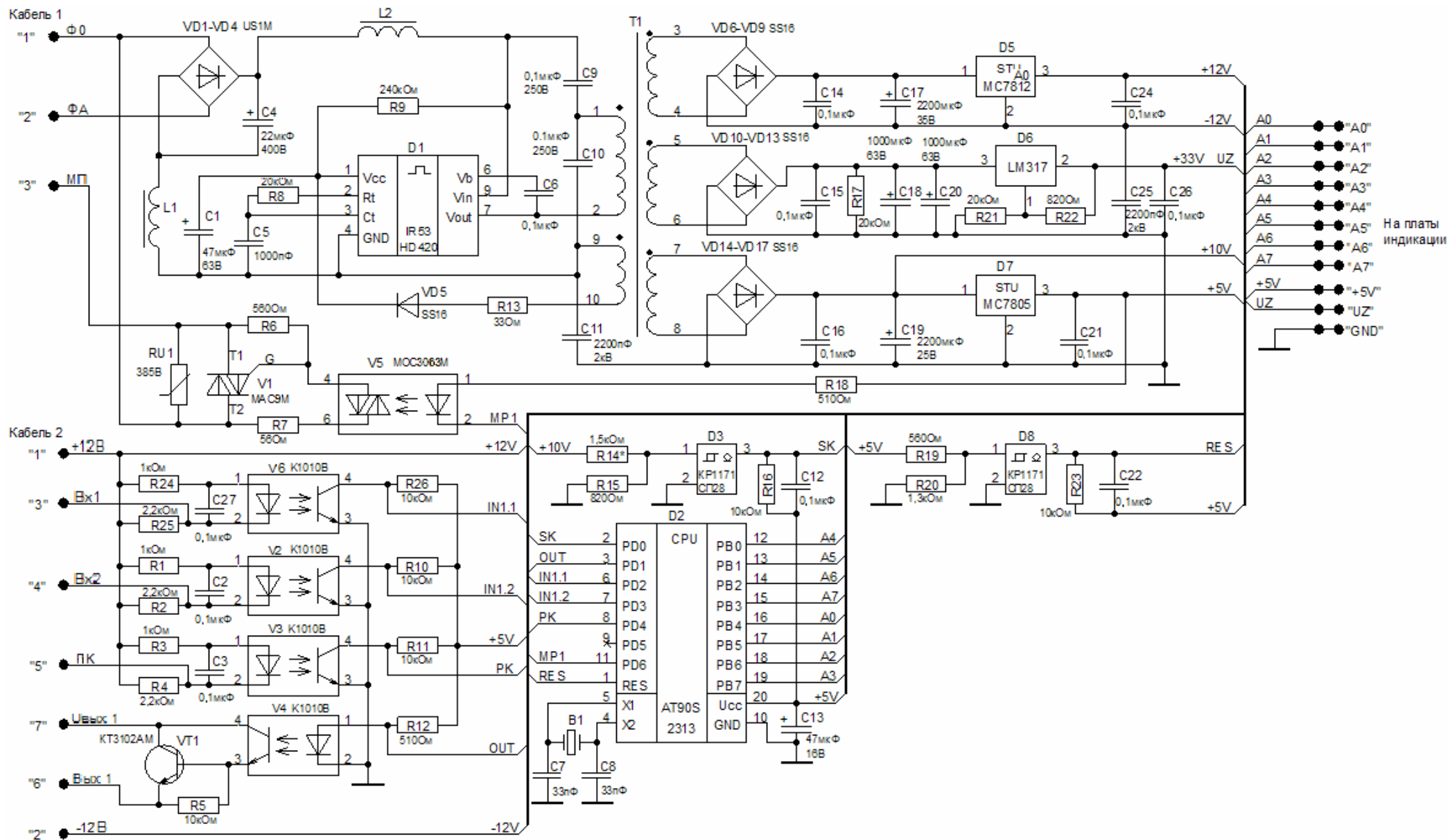
Фрагмент схемы электрической принципиальной устройства отсчетного ЭЦТ 1/5М-5: входные и выходные цепи.
