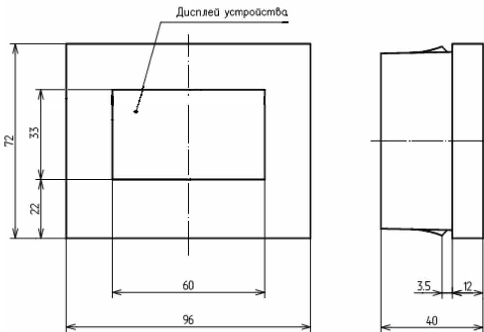
Рисунок А.1. Габаритные размеры устройства
